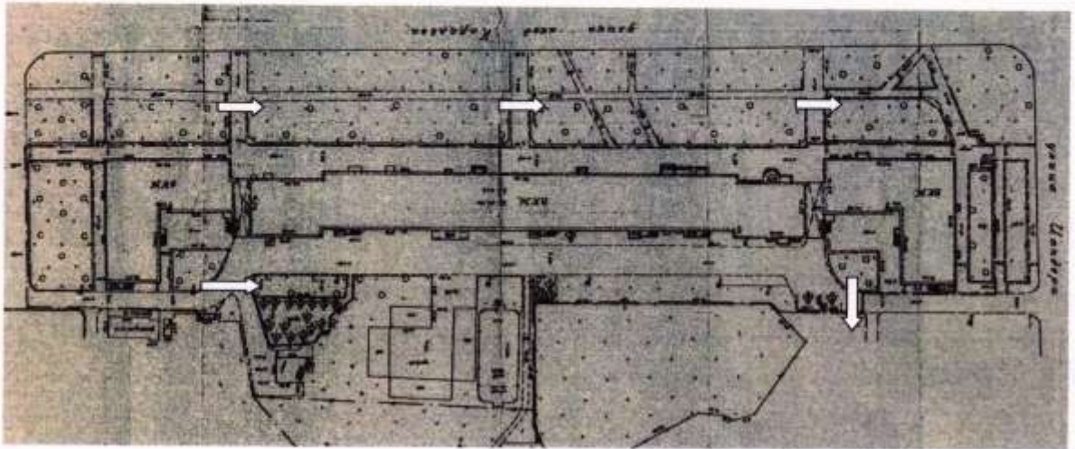
Рис. 1 Схема размещения шлагбаумов
